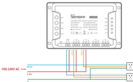
4CHPROR3 (AC Input)
